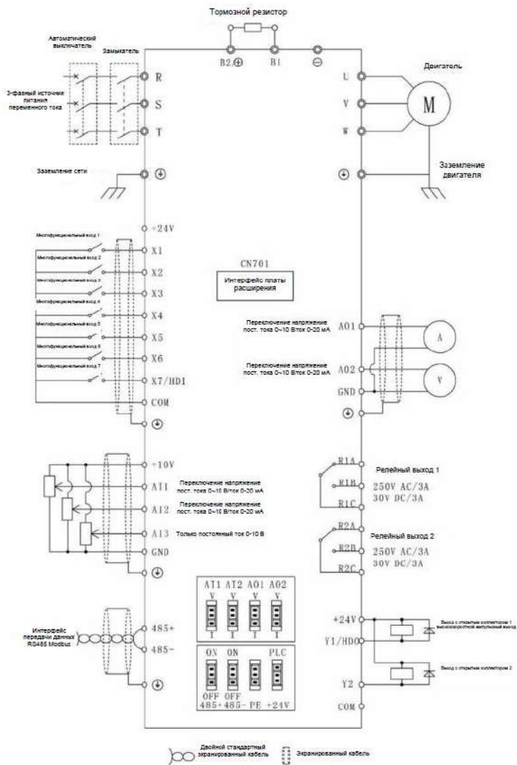
Рис. 2-4 Стандартная схема подключения
