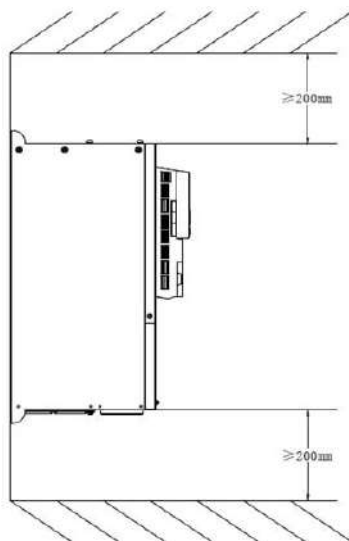
Рис. 2-3 Монтажное положение для преобразователей мощностью от 18,5 кВт
