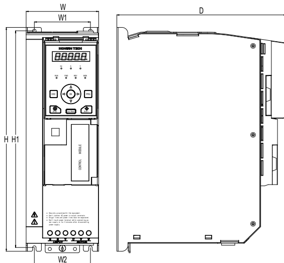
Рис. 1-3 Установочные размеры IMD552U43B (5,5кВт) и ниже
