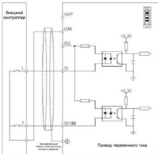
Рис. 2-7 Управление через сухие контакты с использованием внутреннего источника питания
