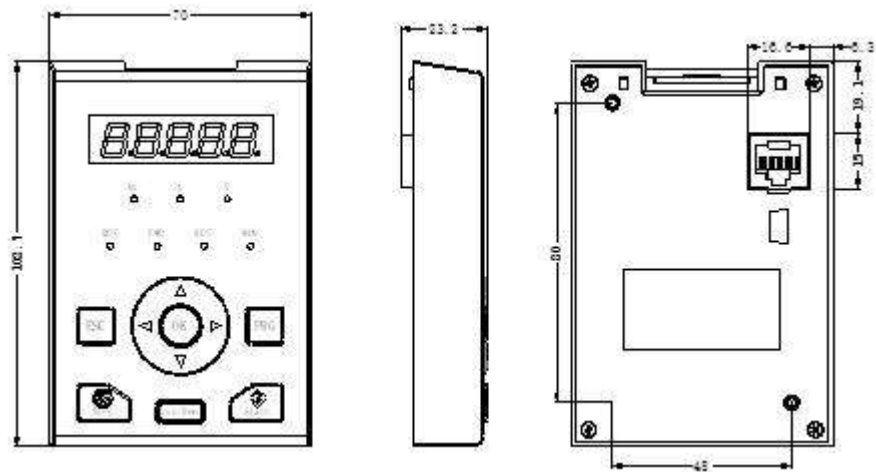
Рис. 1-7 Габаритные размеры панели управления
