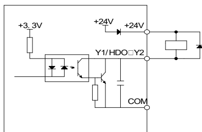
Рис. 2-15 Внутренний источник питания Рис. 2-16 Внешний источник питания
