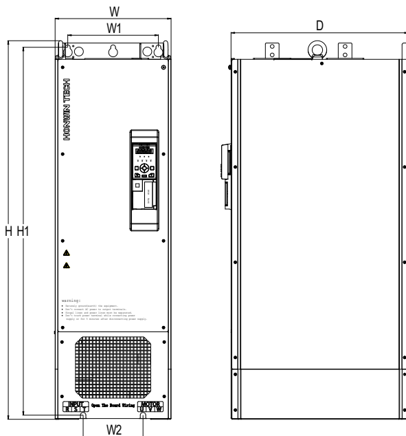
Рис. 1-6 Установочные размеры IMD224U43E~IMD404U43E (220кВт~400кВт)
