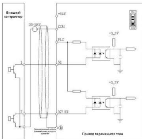
Рис. 2-10 Режим открытого коллектора в режиме NPN с использованием внешнего источника питания
