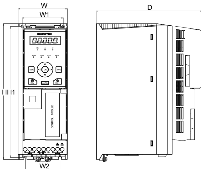
Рис. 1-3 Установочные размеры IMD552U43B (5,5кВт) и ниже
