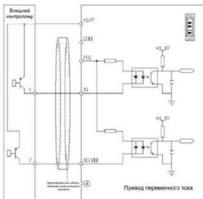
Рис. 2-11 Режим PNP с открытым коллектором при использовании внутреннего источника питания
