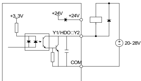
Рис. 2-15 Внутренний источник питания Рис. 2-16 Внешний источник питания
