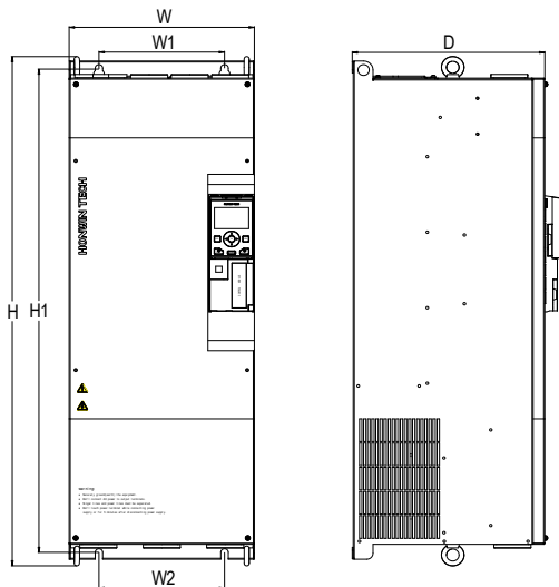
Рис. 1-5 Установочные размеры IMD373U43E~IMD204U43E (37кВт~200кВт)
