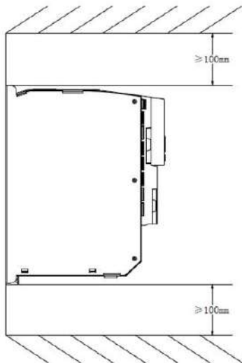
Рис. 2-2 Монтажное положение для преобразователей мощностью до 15 кВт
