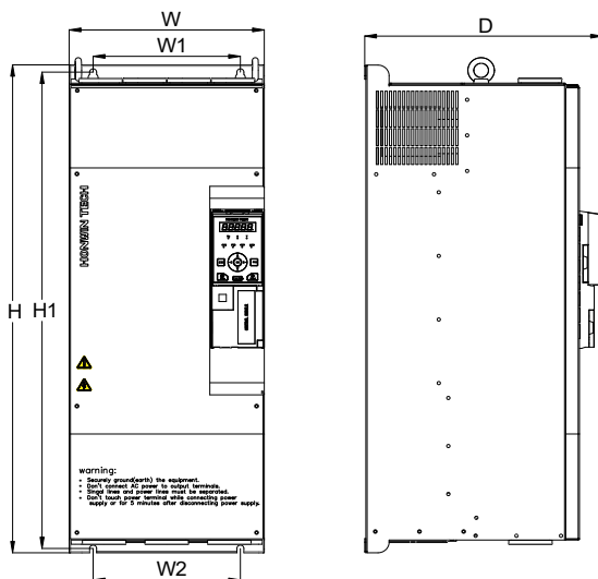
Рис. 1-4 Установочные размеры IMD183U43E~IMD303U43E (18.5кВт~30кВт)
