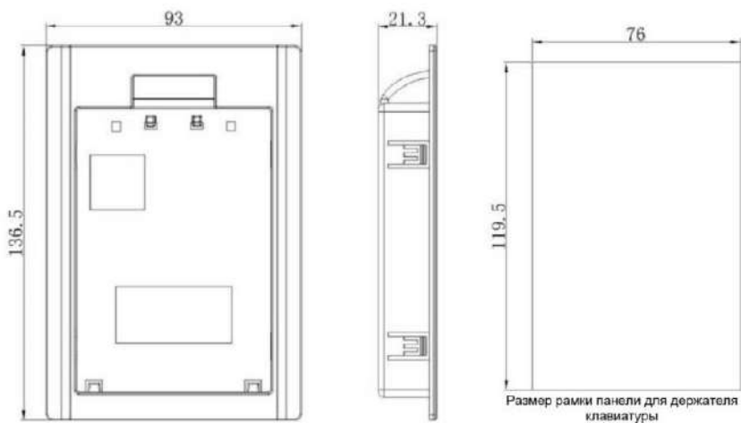
Рис. 1-8 Размеры держателя панели управления
