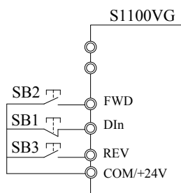
Рисунок 5-9. Трехпроводной режим работы 1
